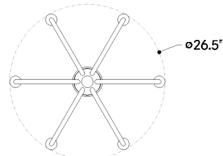
BOTTOM
